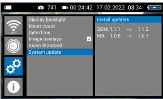
Fig. 36: System-Update
